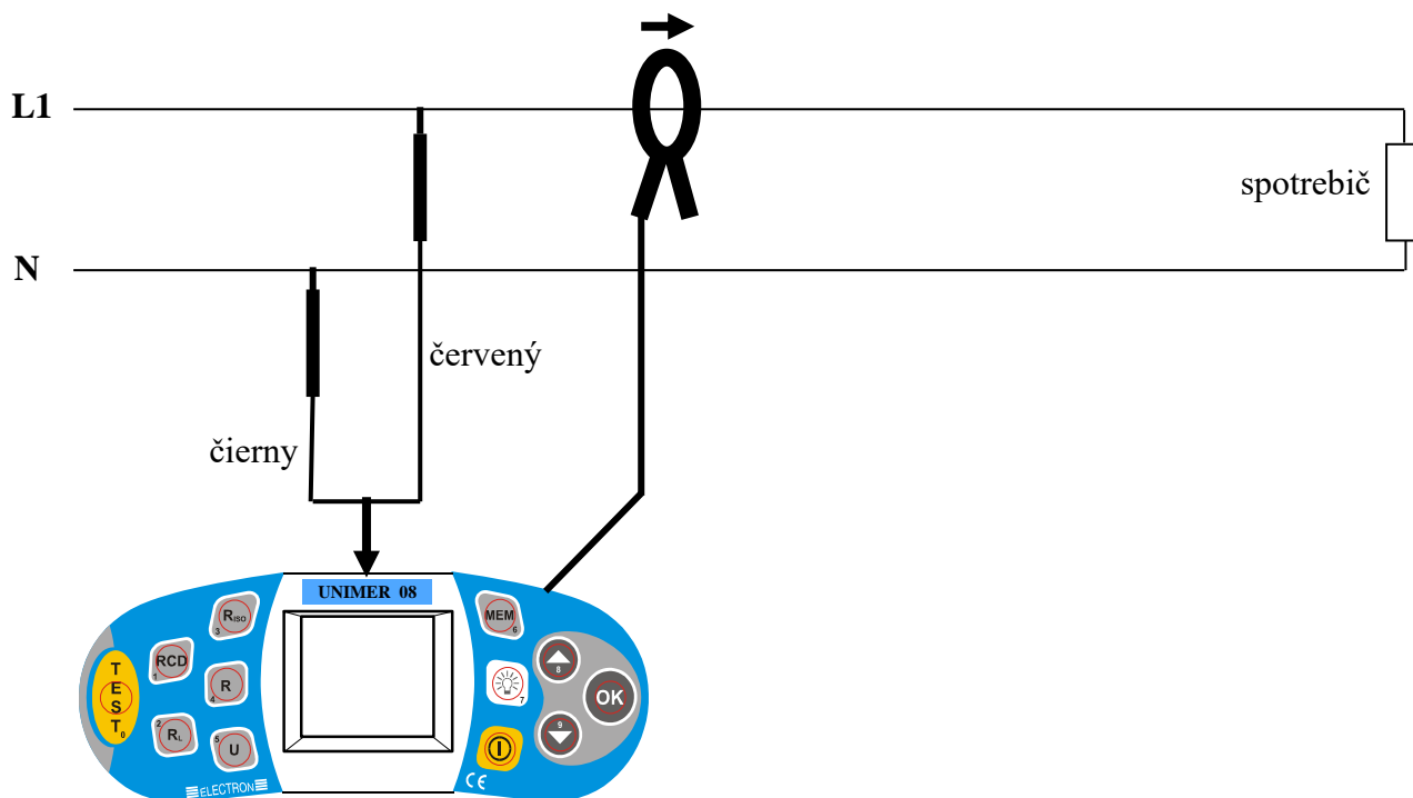
Obr. 6: Meranie príkonu
